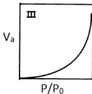
شکل ۹- ایزوترم جذب نوع III
