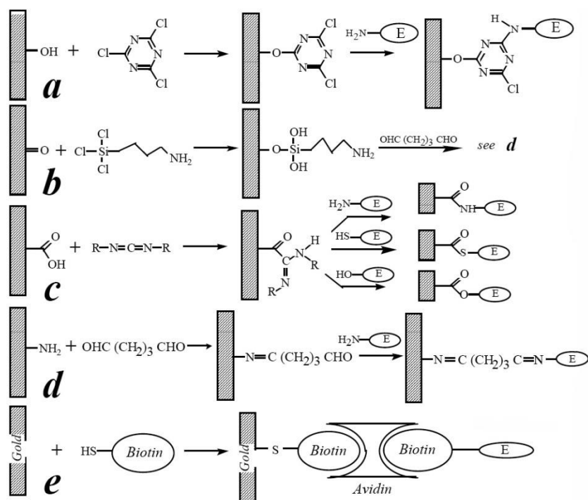
شکل ۴- فعال سازی سطح الکترود برای اتصال به آنزیم [۷]
