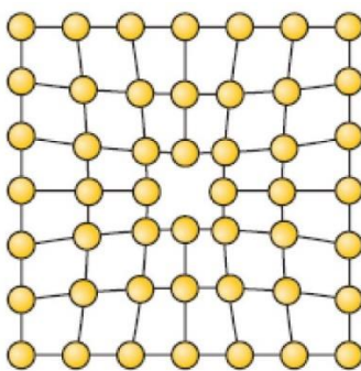
شکل ۲- نمایش جای خالی در یک ساختار بلوری [۲]
