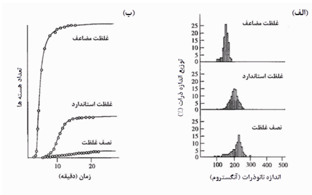
شکل ۲- تاثیر غلظت پیش ماده فلزی بر (الف) تعداد هسته‌های ایجاد شده در زمان‌های مختلف و (ب) توزیع اندازه نانوذرات فلزی سنتز شده با روش احیای شیمیایی
