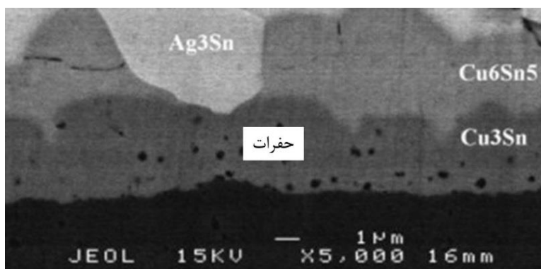
شکل ۱۱- نمایش حفرات (عیب سه‌بعدی) در تصویر SEM
