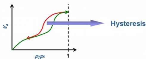
شکل ۱۳- هیسترسیس جذب و واجذب [۱۳].
