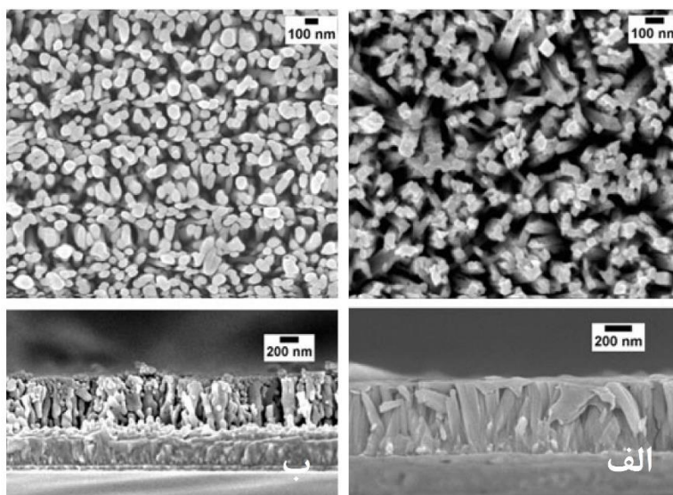
شکل ۷- تصاویر میکروسکوپ الکترونی روبشی از سطح خارجی و سطح مقطع نانوسیم های آمورف \text{FeOOH} قبل از تکلیس (الف) و نانوسیم های \text{FeOOH} بلوری بعد از فرآیند تکلیس (ب)
