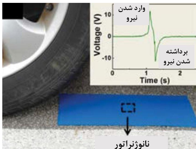
شکل ۸- استفاده از نانوسیم‌های اکسید روی به عنوان نانوژنراتور برای تولید الکتریسیته از حرکت خودروها بر روی صفحه نانوژنراتور [۸]
