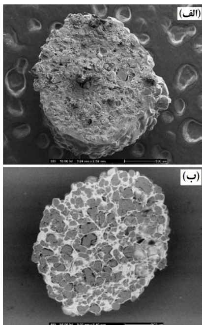
شکل ۷- تصویر الف-SE و ب- BSE از سطح مقطع یک ذره. SE برای تصویربردای در حالت توپوگرافی و مورفولوژی و BSE برای کنتراست توزیع فازی مناسب است
