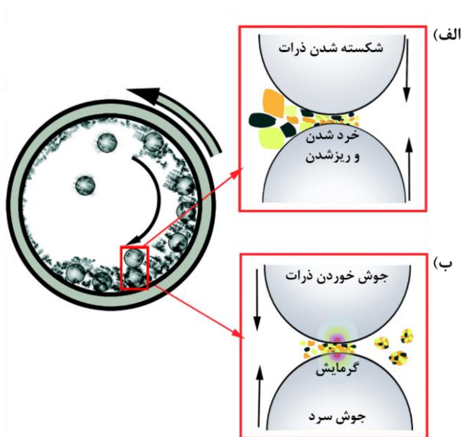
شکل ۳: شکستن و جوش خوردن ذرات در فرایند آسیاب کاری. (DOI: ۱۰.۱۰۳۹/C5CE۰۰۱۲۳K)
