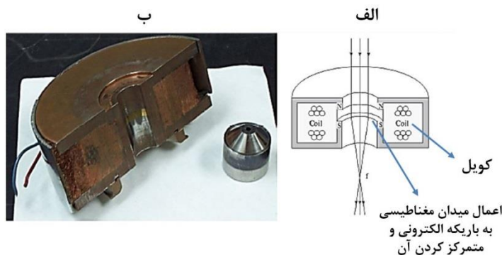
شکل ۴- الف) تصویر نحوه عملکرد عدسی الکترومغناطیسی و ب) تصویر واقعی یک عدسی الکترومغناطیسی
