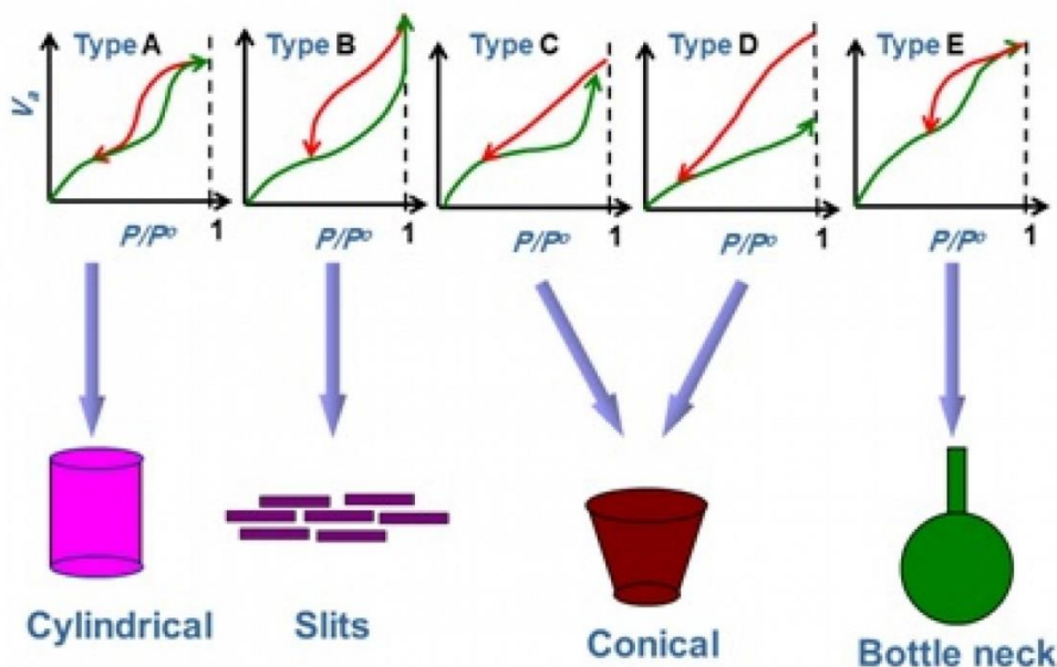
شکل ۱۴- انواع هیستریسیس با توجه به هندسه حفره [۲].
