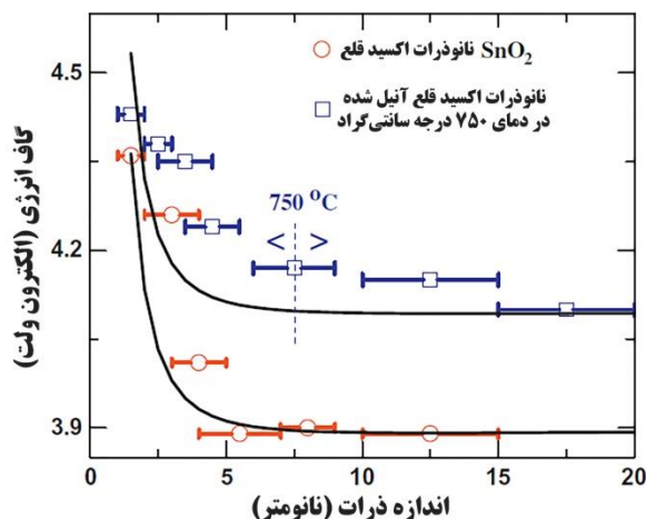
شکل ۸- تغییرات گاف انرژی اکسیدقلع با اندازه نانوذرات [۶]
