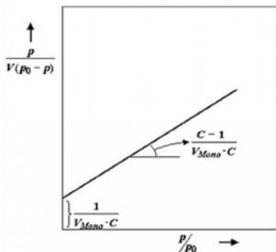
شکل ۵- نمودار BET [۱۱].
